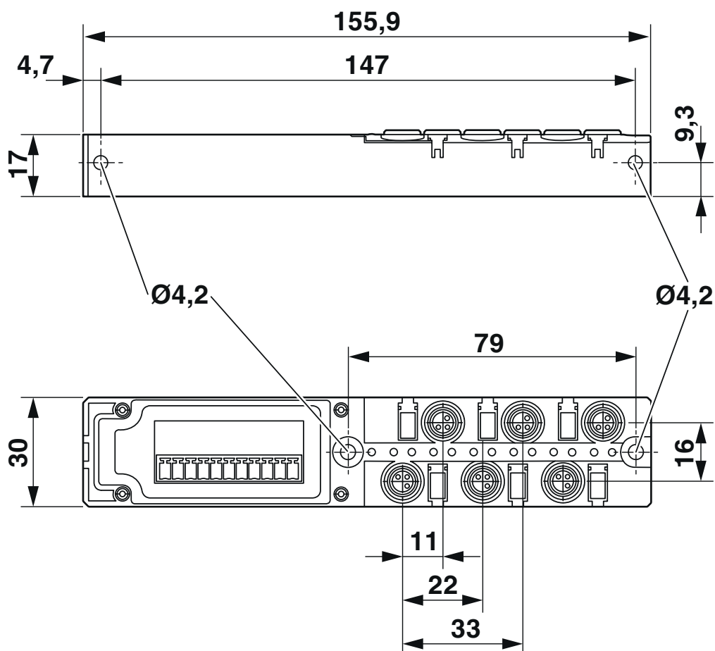
Maßzeichnung
