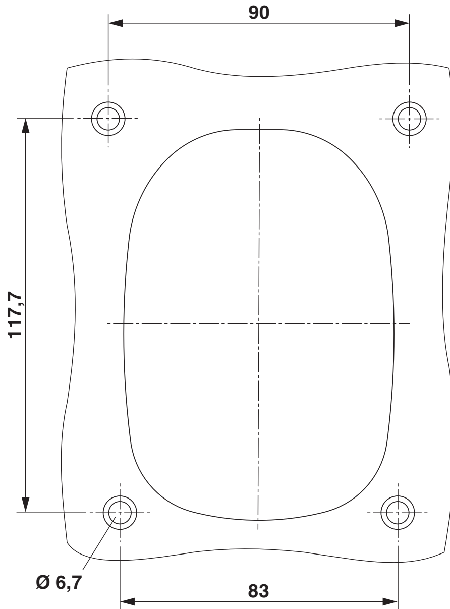
Bohrplan/Lötpadgeometrie
