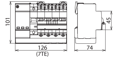
Maßbild SPD+POP 4 255 C40
