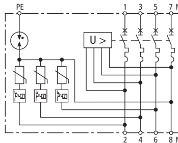
Prinzipialschaltbild SPD+POP 4 255 C40
