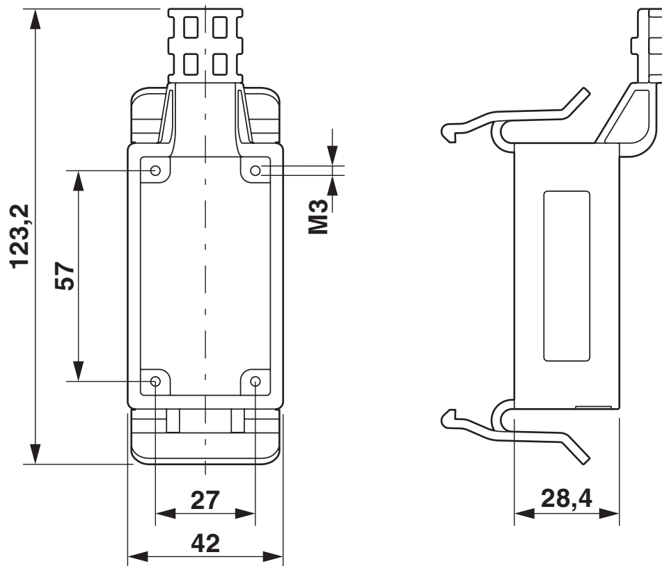
Maßzeichnung
