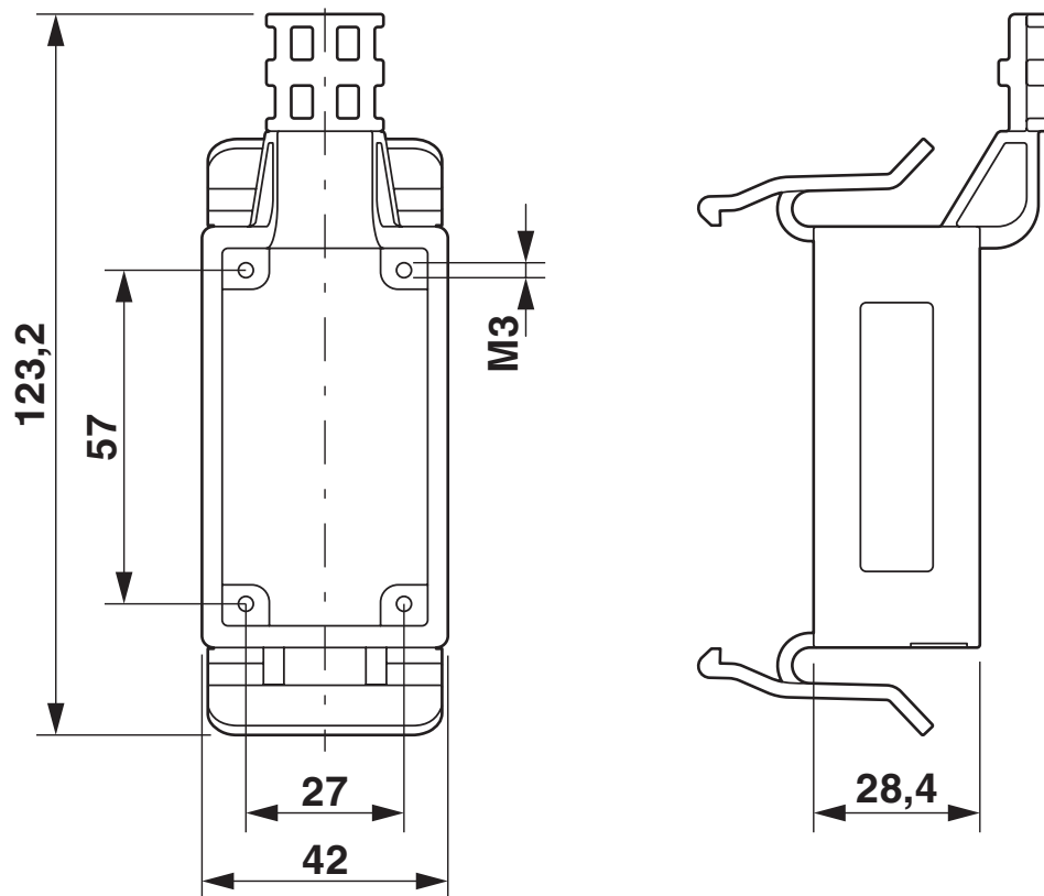
Dessin coté
