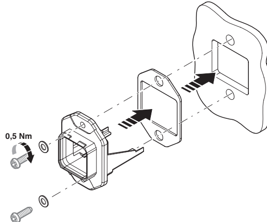
Explosionszeichnung
