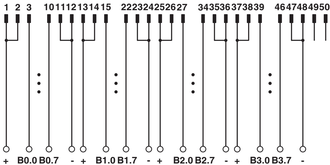
Esquema de conexiones VIP-2/.../FLK50/PLC
