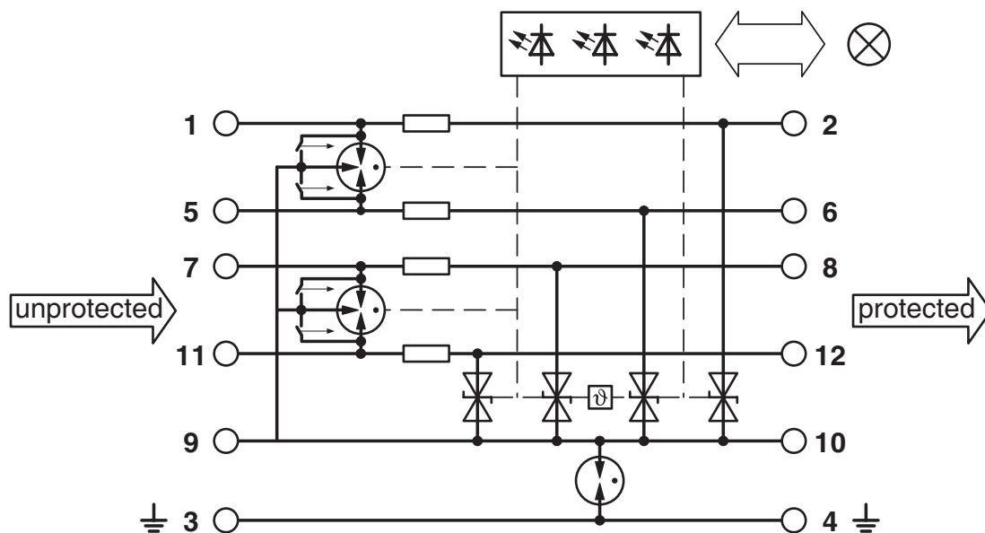
Diagrama eléctrico
