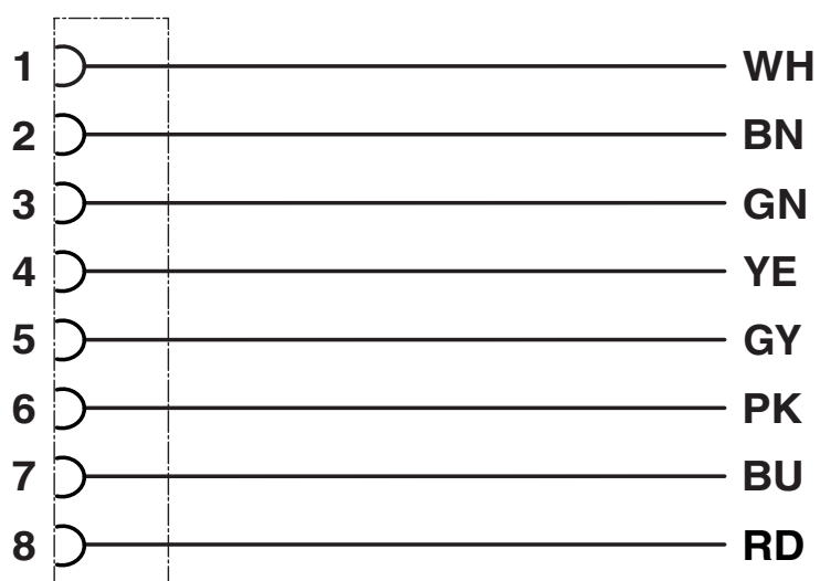
Diagrama eléctrico
