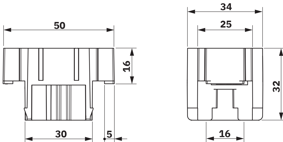
Dessin coté
