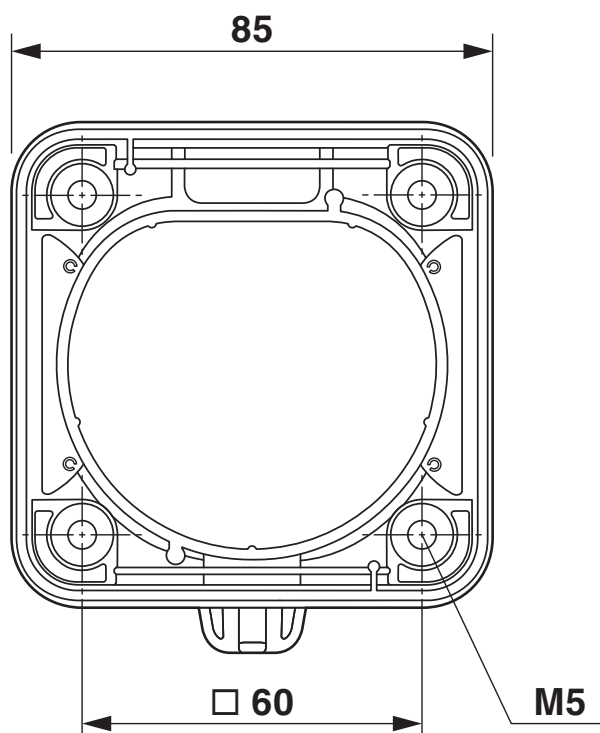
Dessin coté
