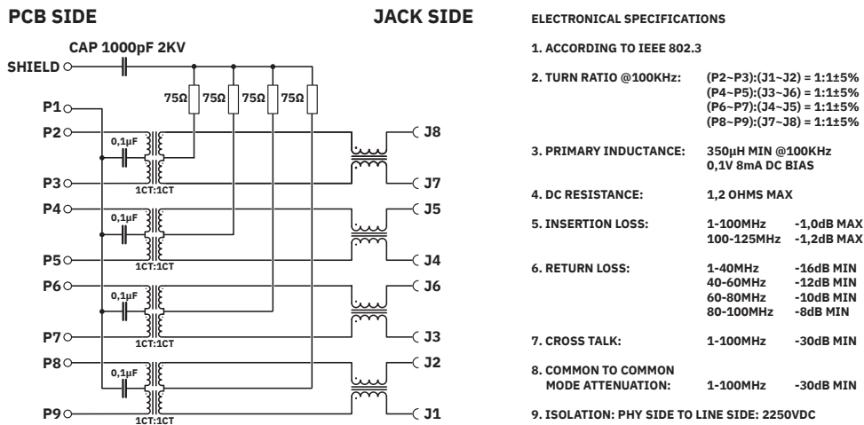
Diagrama eléctrico
