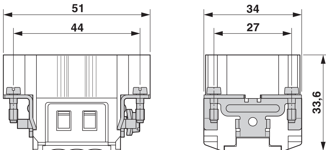
Maßzeichnung
