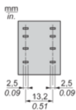
Stecker-Seitenansicht
