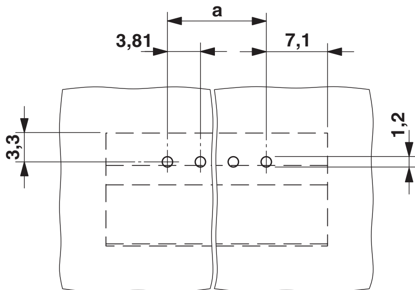
Bohrplan/Lötpadgeometrie
