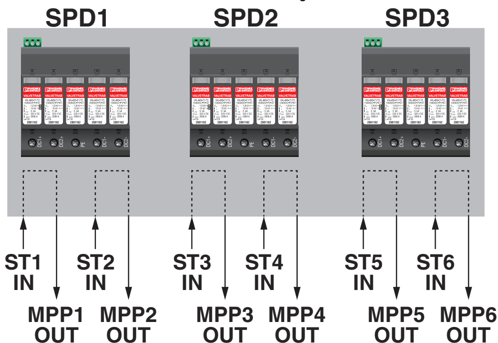
Anschlusszeichnung
