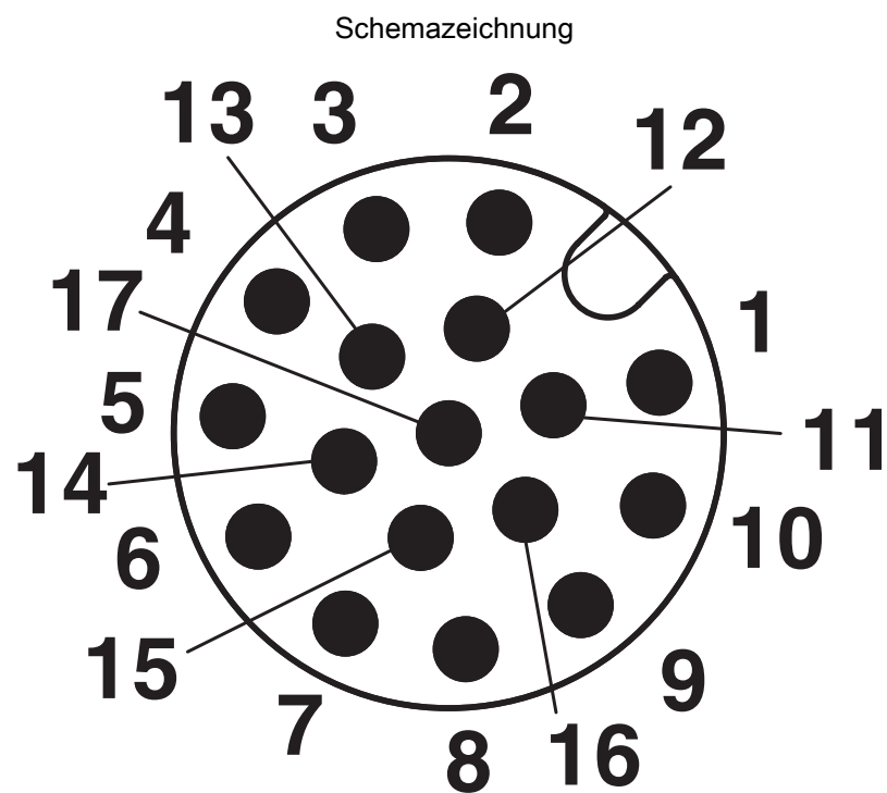
Polbild M12-Stecker, 17-polig, Ansicht Stiftseite
