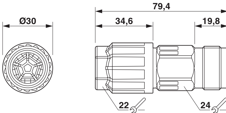
Maßzeichnung
