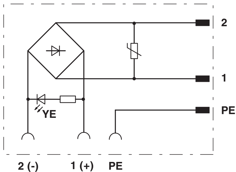
Diagrama eléctrico
