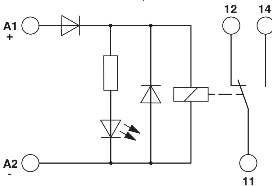
Schaltplan
