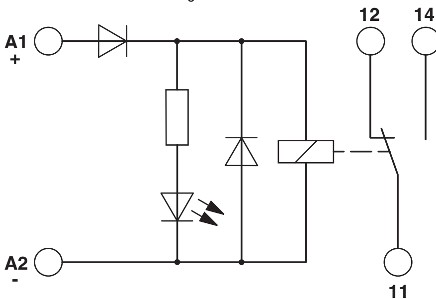
Diagrama eléctrico
