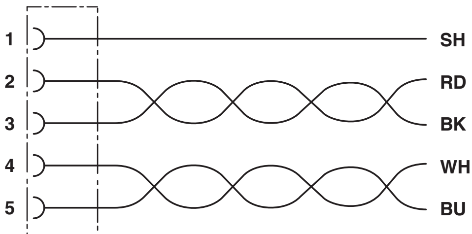
Ocupación de contactos del conector hembra M12
