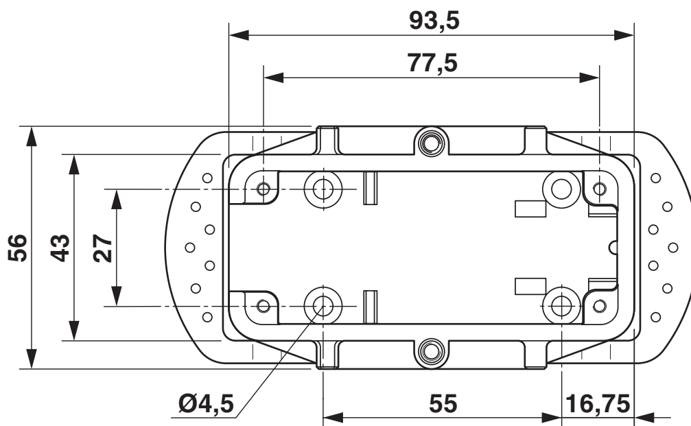
Esquema dimensiones vista desde arriba
