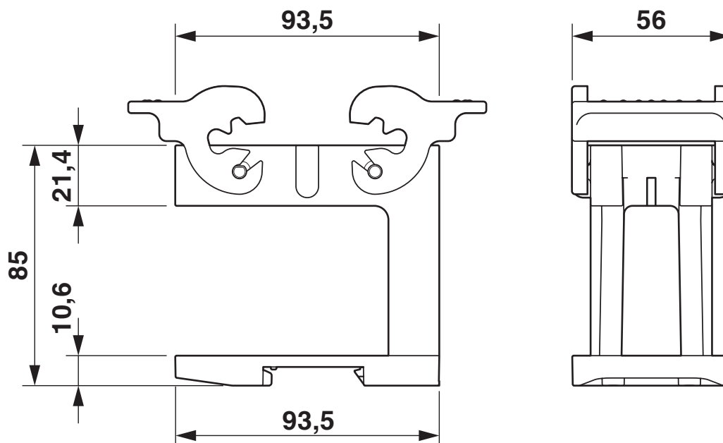
Dessin coté
