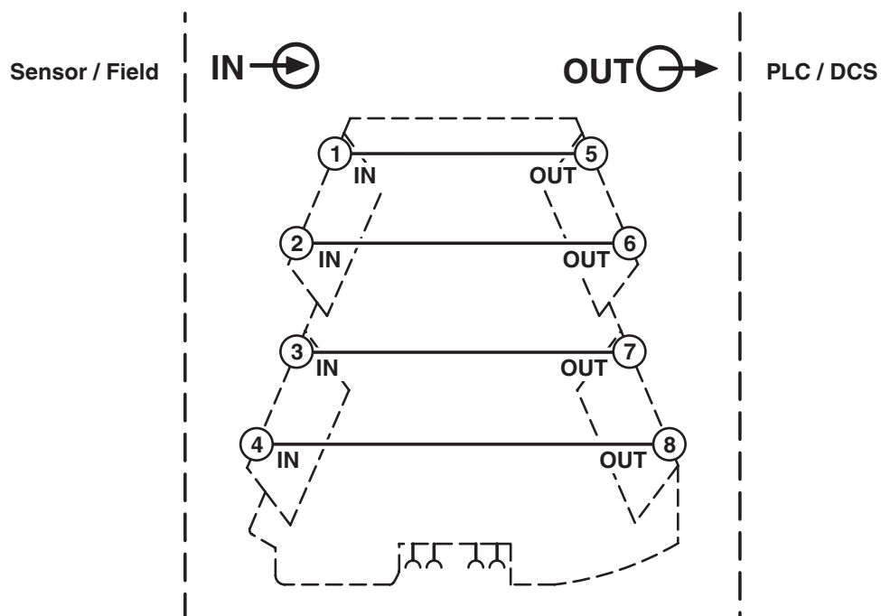
Schéma fonctionnel
