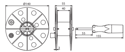
Maßbild DH K 40 BS ML0.75 L50M BL
