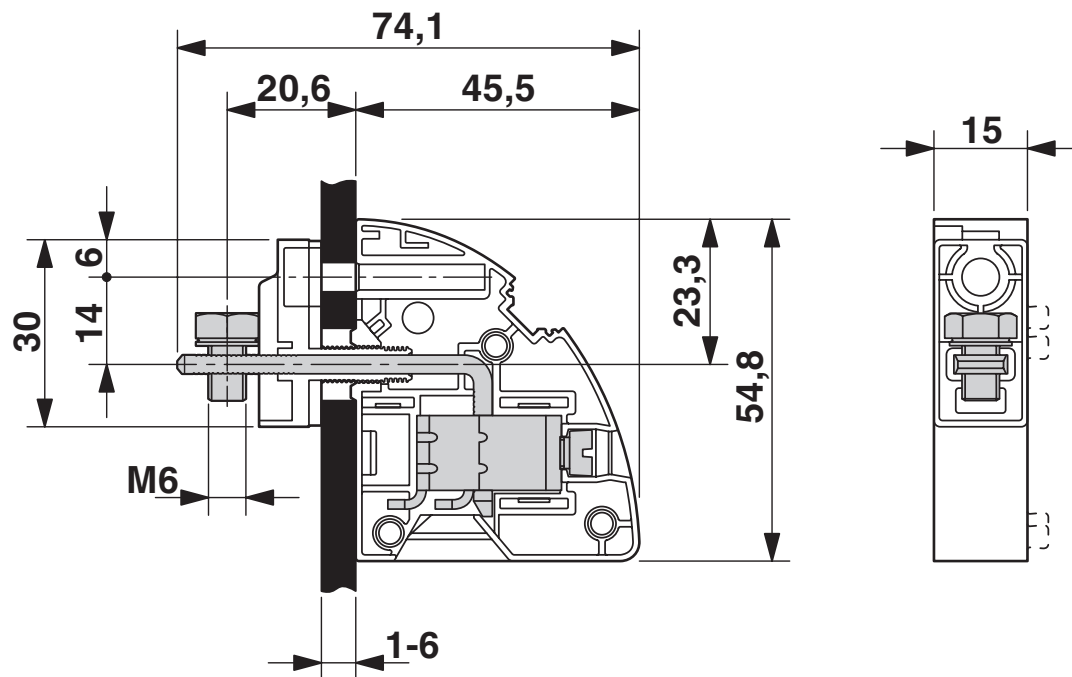
Dessin coté
