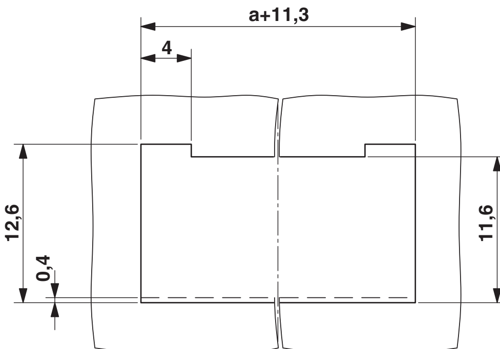
Schemazeichnung
