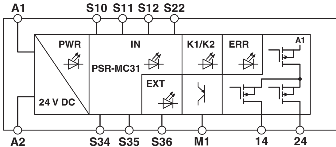
Schéma fonctionnel
