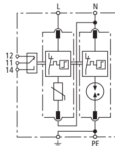
Prinzipschaltbild DG M TT 2P 385 FM
