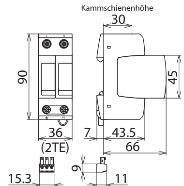
Maßbild DG M TT 2P 385 FM
