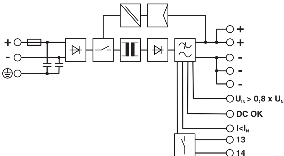
Schéma fonctionnel
