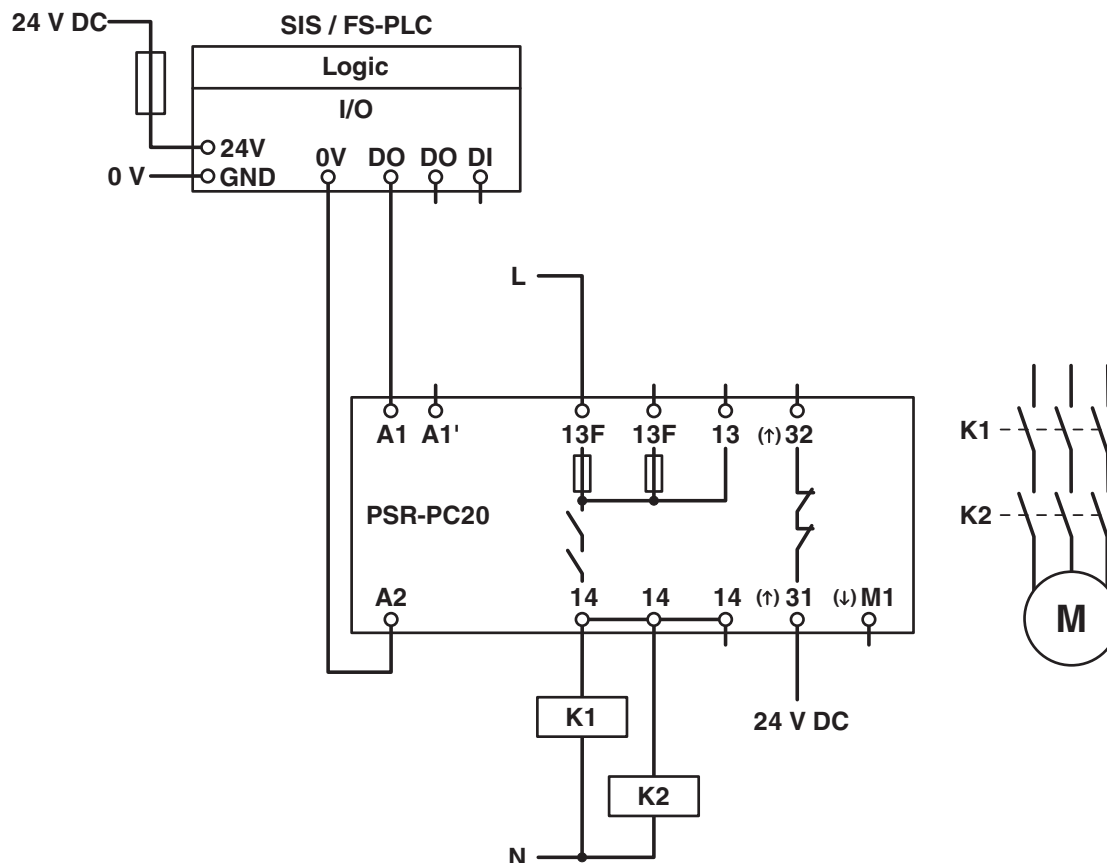
Diagrama eléctrico
