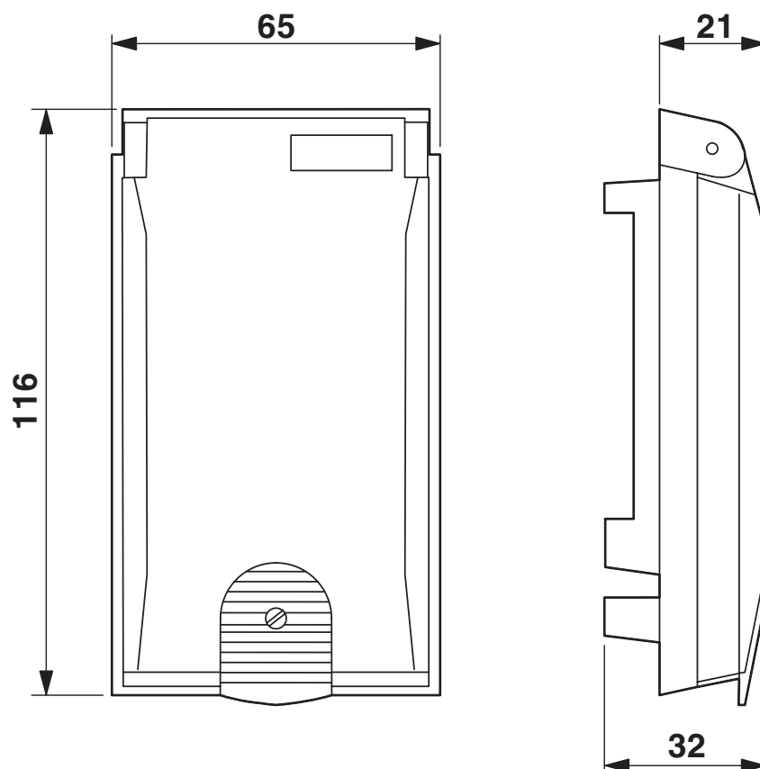
Dessin coté
