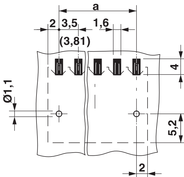
Bohrplan/Lötpadgeometrie
