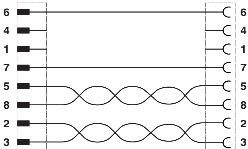
Diagrama eléctrico
