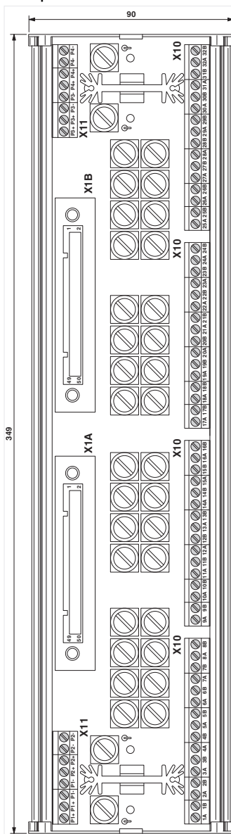
Esquema de dimensiones
