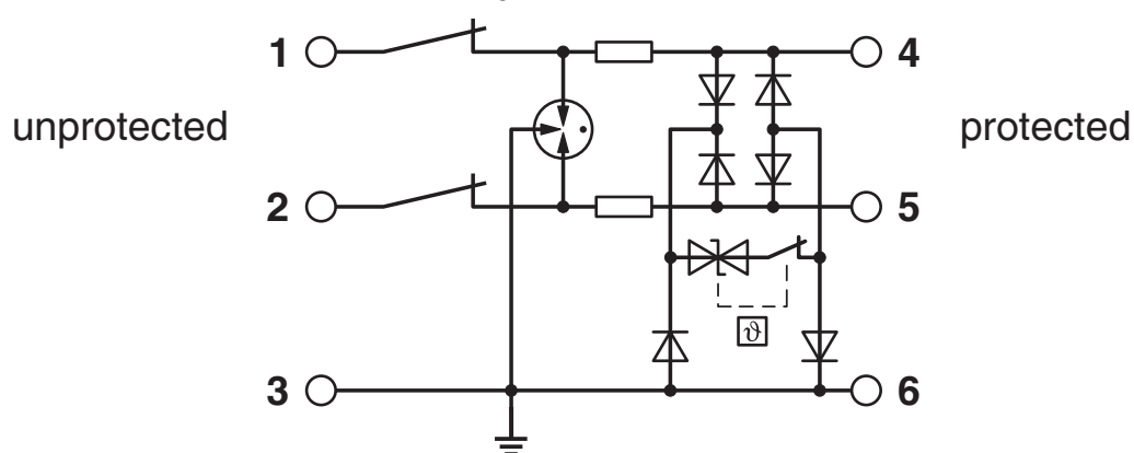
Diagrama eléctrico
