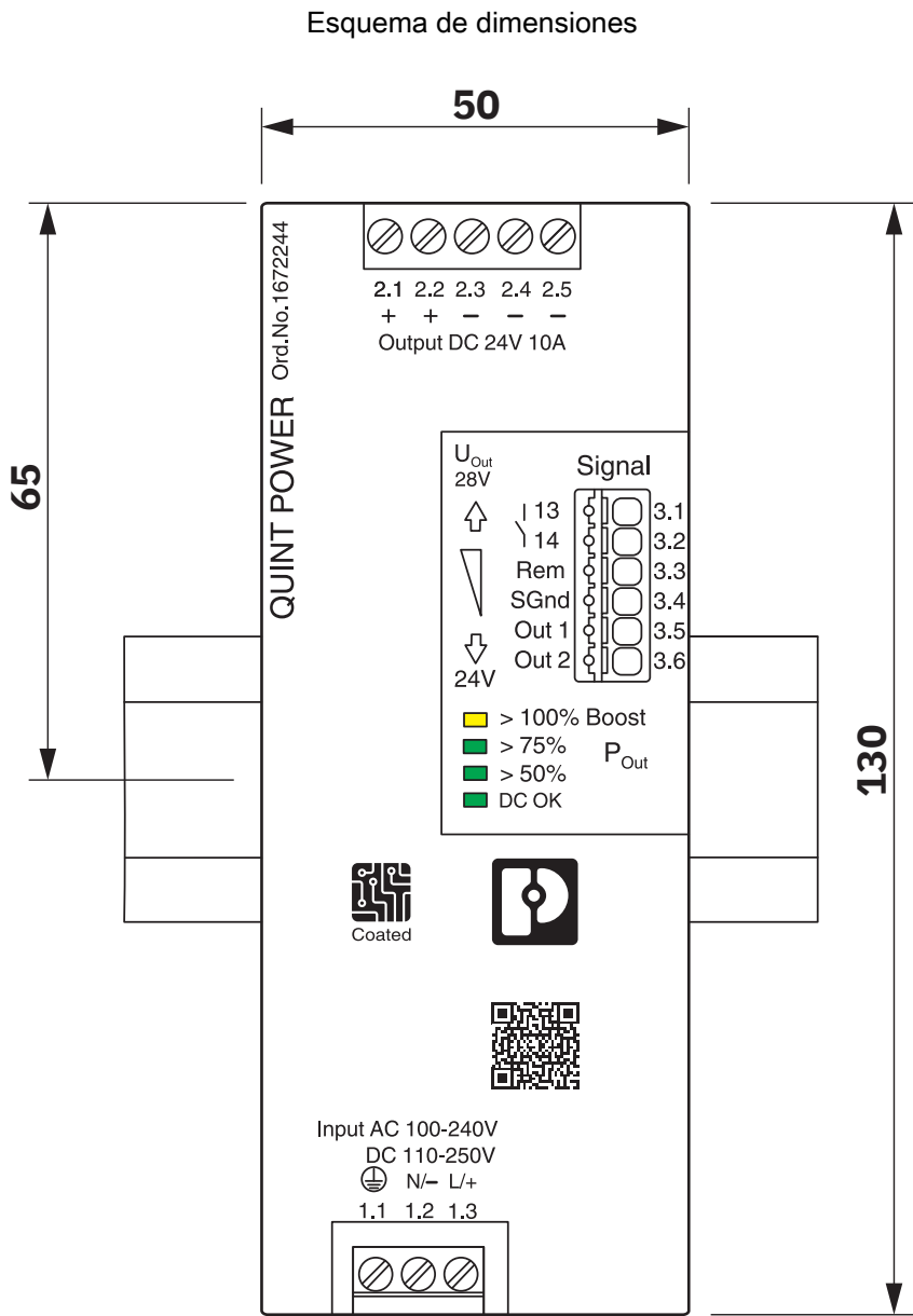
Dimensiones del dispositivo (medidas en mm)
