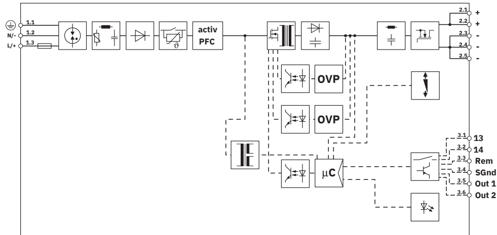
Schéma fonctionnel
