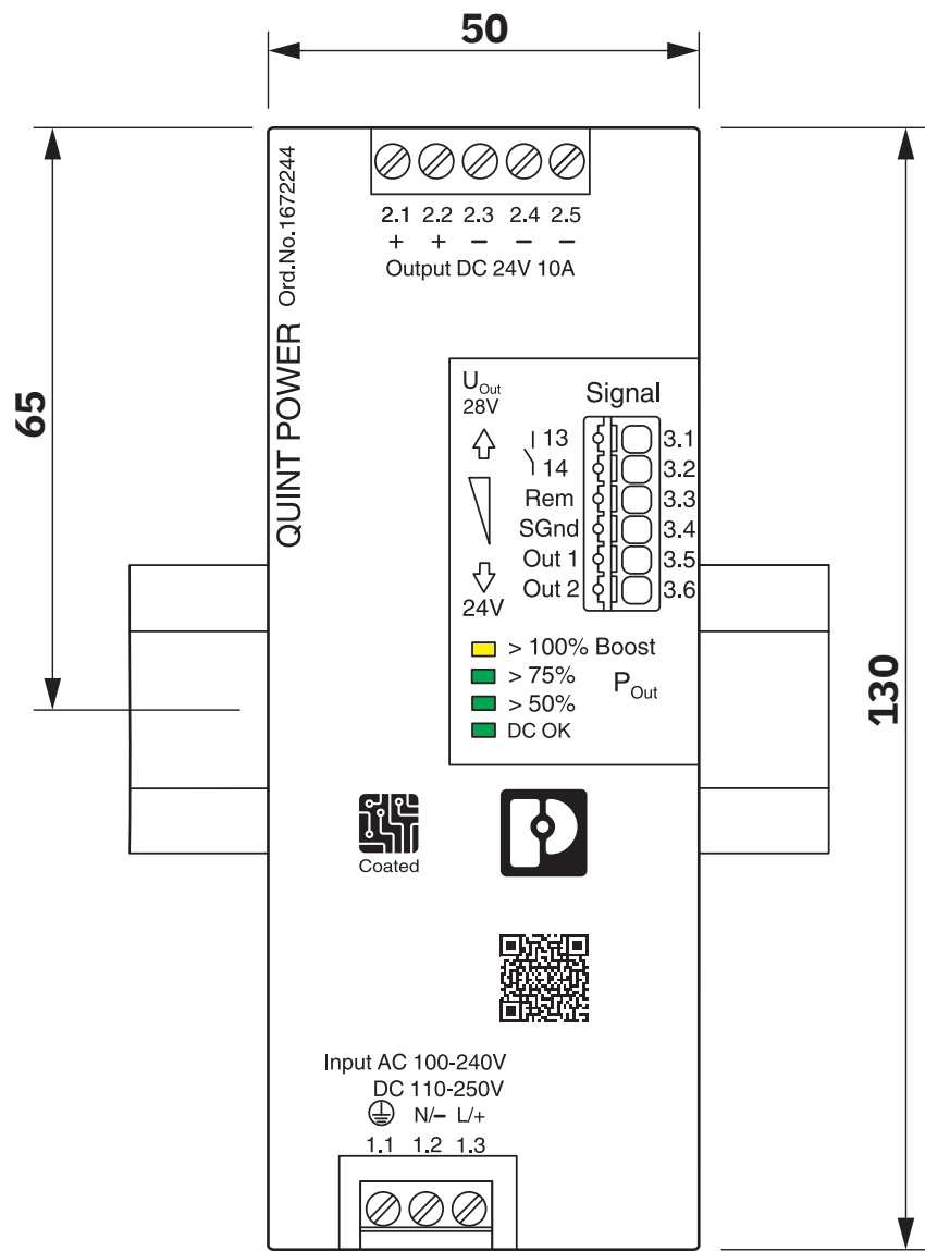
Encombrement de l'appareil (cotes en mm)
