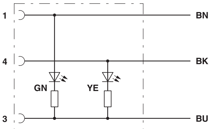
Disposition des contacts des connecteurs femelles M8/M12 avec 2 LED
