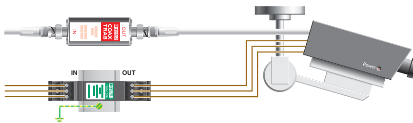
Applikationszeichnung
