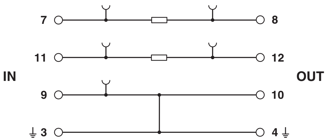
Schaltplan
