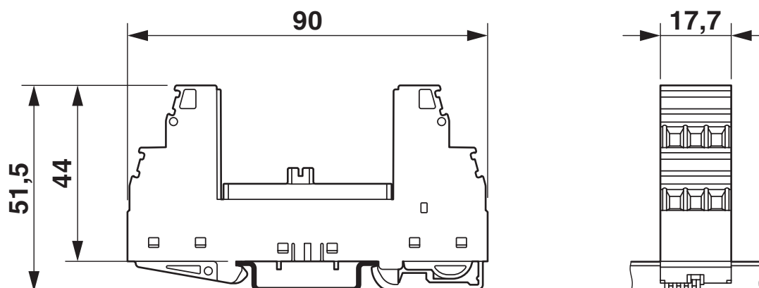
Dessin coté
