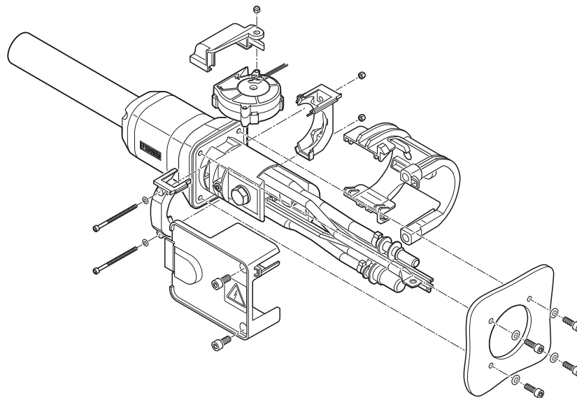
Montageanleitung zur Anbringung des Berührschutzes am Beispiel der geraden Wanddurchführung
