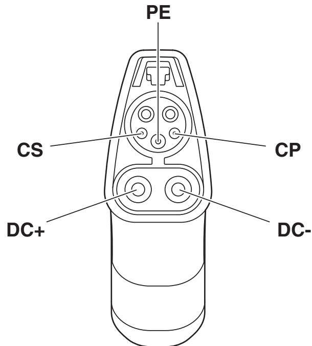
Schemazeichnung
