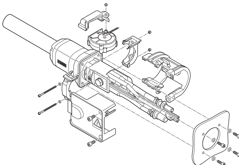
Instructions de montage pour la mise en place de la protection contre les contacts, exemple de la traversée de paroi droite
