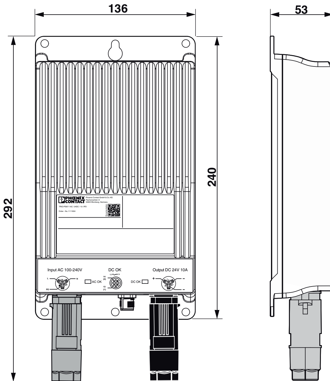
Maßzeichnung
