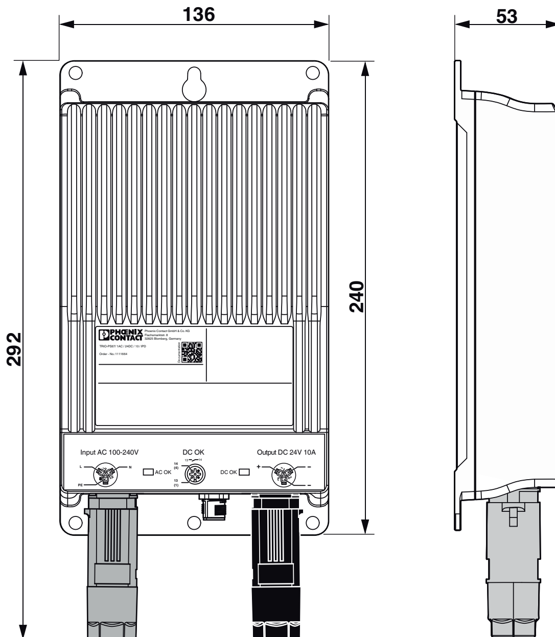
Dessin coté
