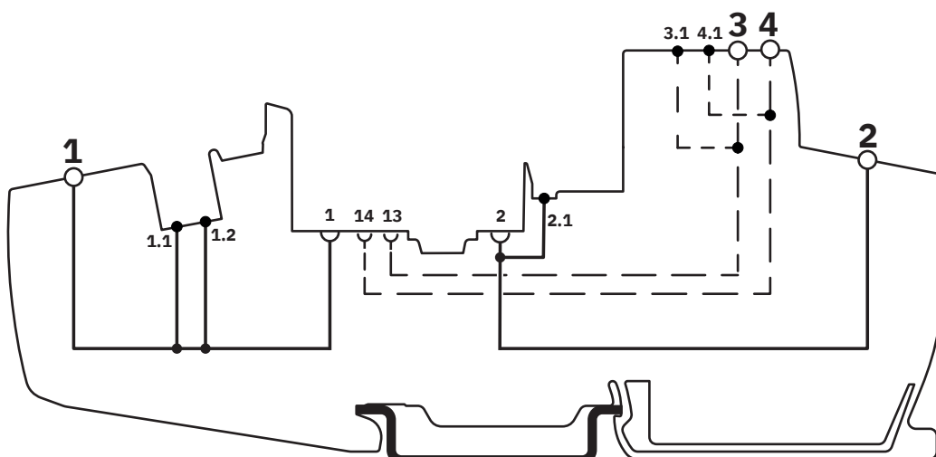
Anschlusszeichnung
