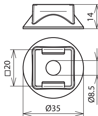
Maßbild KS 35 14 B8.5 UVS GR
