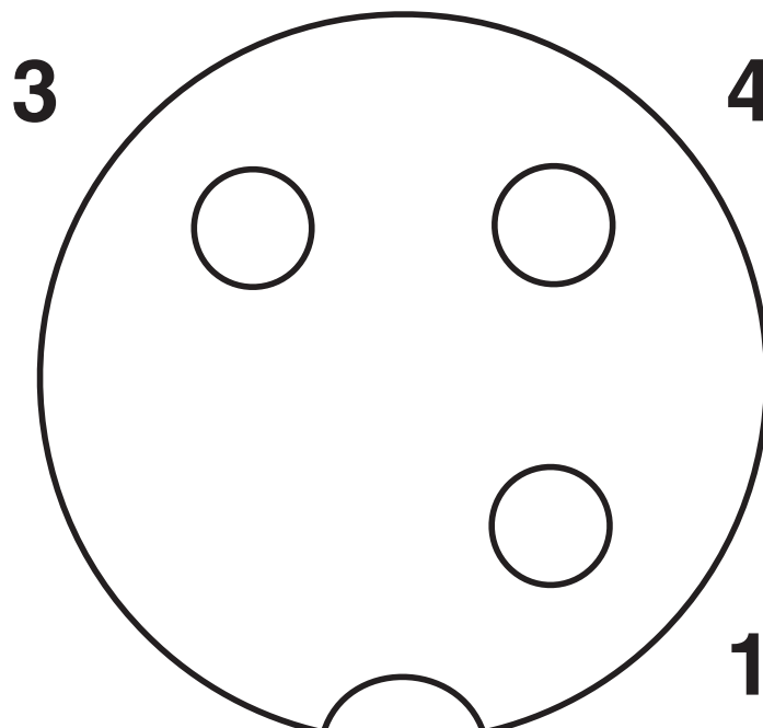
Schemazeichnung
