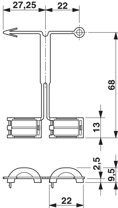
Dessin coté
